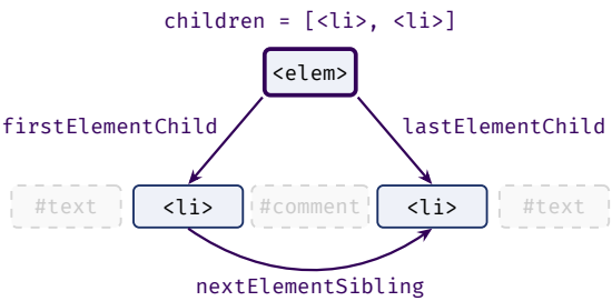
Gli stessi nodi della figura precedente: i nodi grigi vengono scavalcati.
