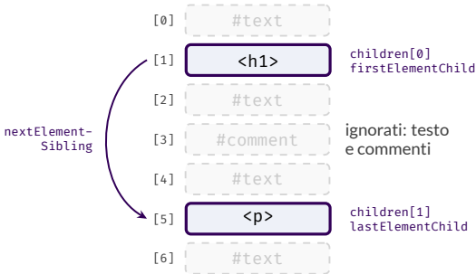
I sette childNodes di <main> : per children contano solo i due elementi.
