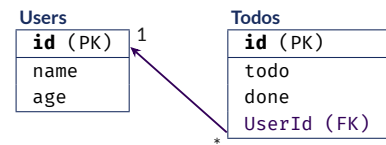
Uno-a-molti: la chiave esterna UserId sta nella tabella dei Todos .
