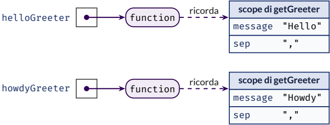
Ogni chiamata a getGreeter crea uno scope nuovo, e la funzione restituita lo porta con sé.
