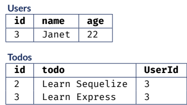
Una sola chiamata, tre righe in due tabelle.
