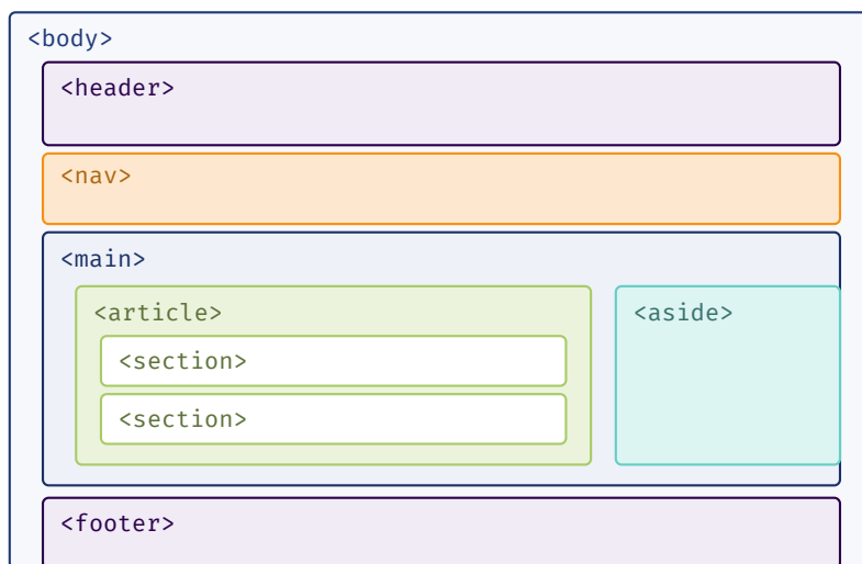
Figura 2.7: Un tipico impianto di pagina realizzato con tag semantici.
