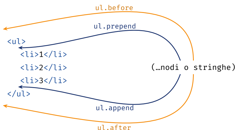
Figura 7.5: I quattro punti di inserimento rispetto alla lista ul : in blu dentro la lista, in arancione fuori , accanto a essa.
