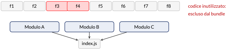
Figura 17.2: Il tree shaking esclude dal bundle il codice mai raggiunto.
