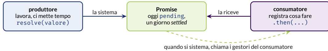
Figura 8.1: La Promise sta fra chi produce un risultato e chi lo usa: nessuno dei due deve aspettare l'altro.
