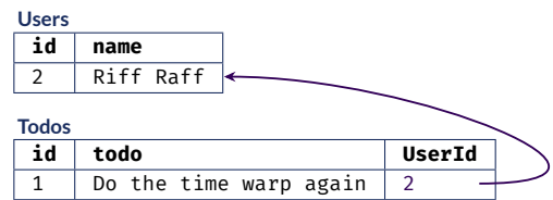
Il todo punta all'utente tramite UserId .
