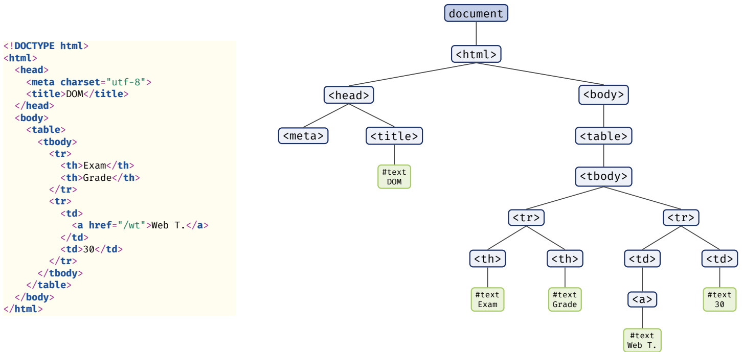
Figura 7.2: Un documento HTML e il corrispondente albero DOM: in blu gli elementi, in verde i nodi di testo.
