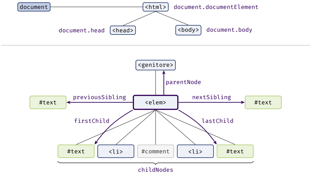
Figura 7.3: In alto, le scorciatoie per gli elementi più esterni. In basso, i riferimenti che ogni nodo ha verso genitore, fratelli e figli: i fratelli e i figli possono essere anche nodi di testo e commenti.
