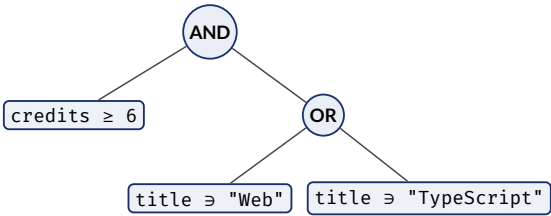
La condizione del filtro come albero: la stessa del WHERE in SQL.
