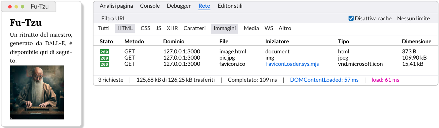
Figura 2.9: La scheda Rete di Firefox durante il caricamento di image.html : tre richieste per una sola pagina.
