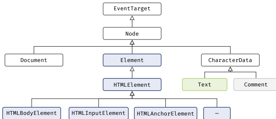
Figura 7.4: La gerarchia delle interfacce del DOM. La freccia con il triangolo vuoto (la generalizzazione di UML) si legge «è un tipo particolare di».
