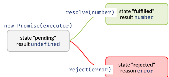
Il ciclo di vita di una Promise.
